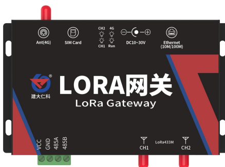
RS-LG-200 LORA 网关
