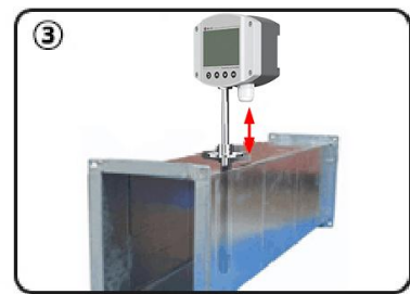
将设备插入到法兰盘中，完成安装
