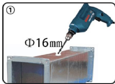
在排风管上打一个直径16mm的孔
