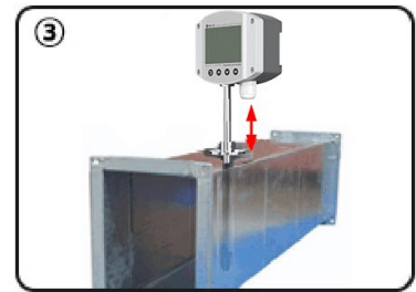
将设备插入到法兰盘中，完成安装
