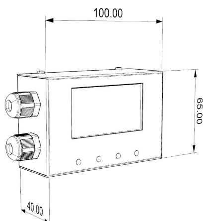
设备尺寸图（单位：mm）
