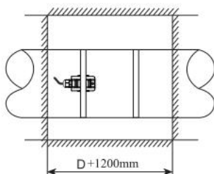
注：D代表管道直径
