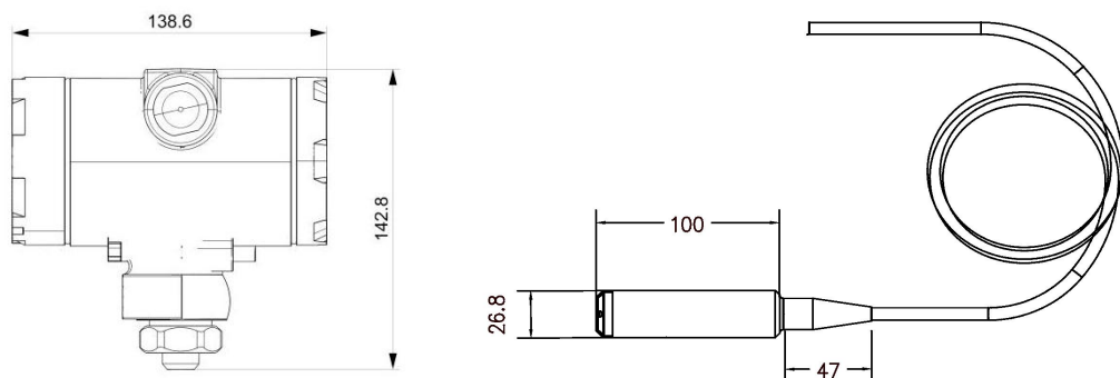
尺寸图 (单位: mm)
