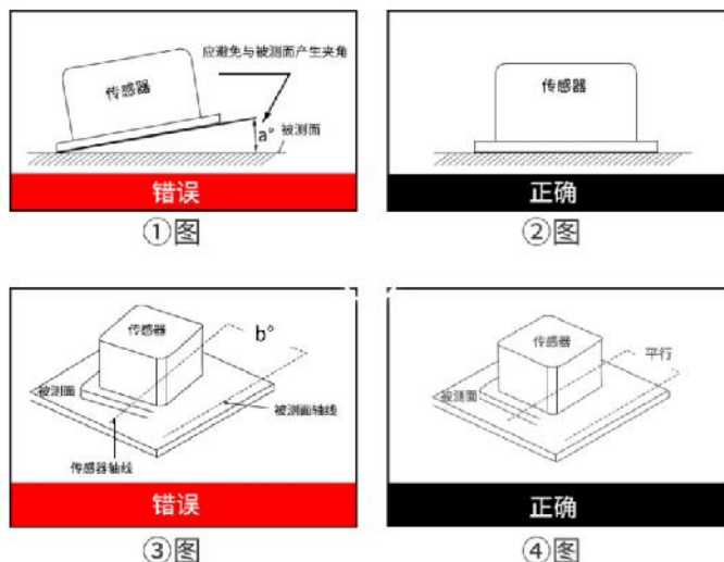
安装示意图
