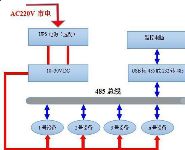
系统方案图
