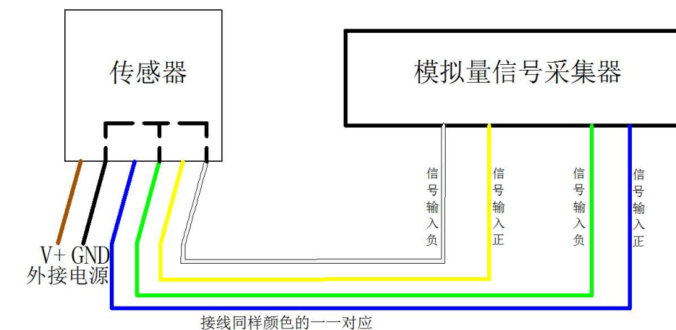
四线制接线示意图
