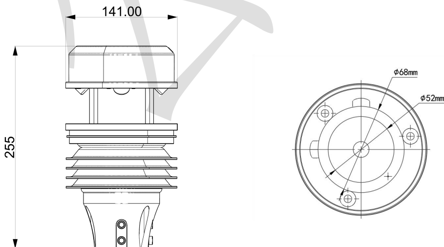
-2H 及-2HS 设备尺寸图（单位：mm）
