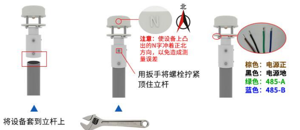
-2 选型安装方式
