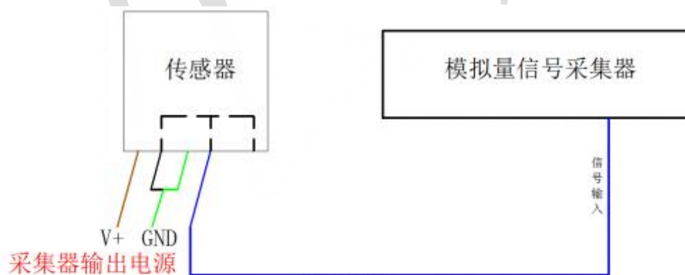
三线制接法示意图
