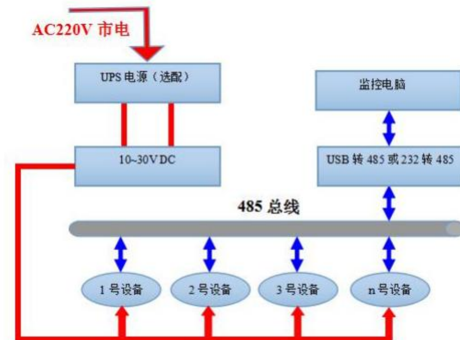
系统方案框图
