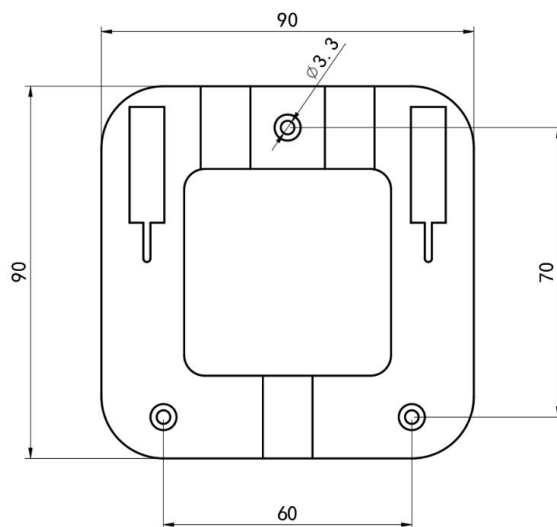
安装底座尺寸（单位：mm）
