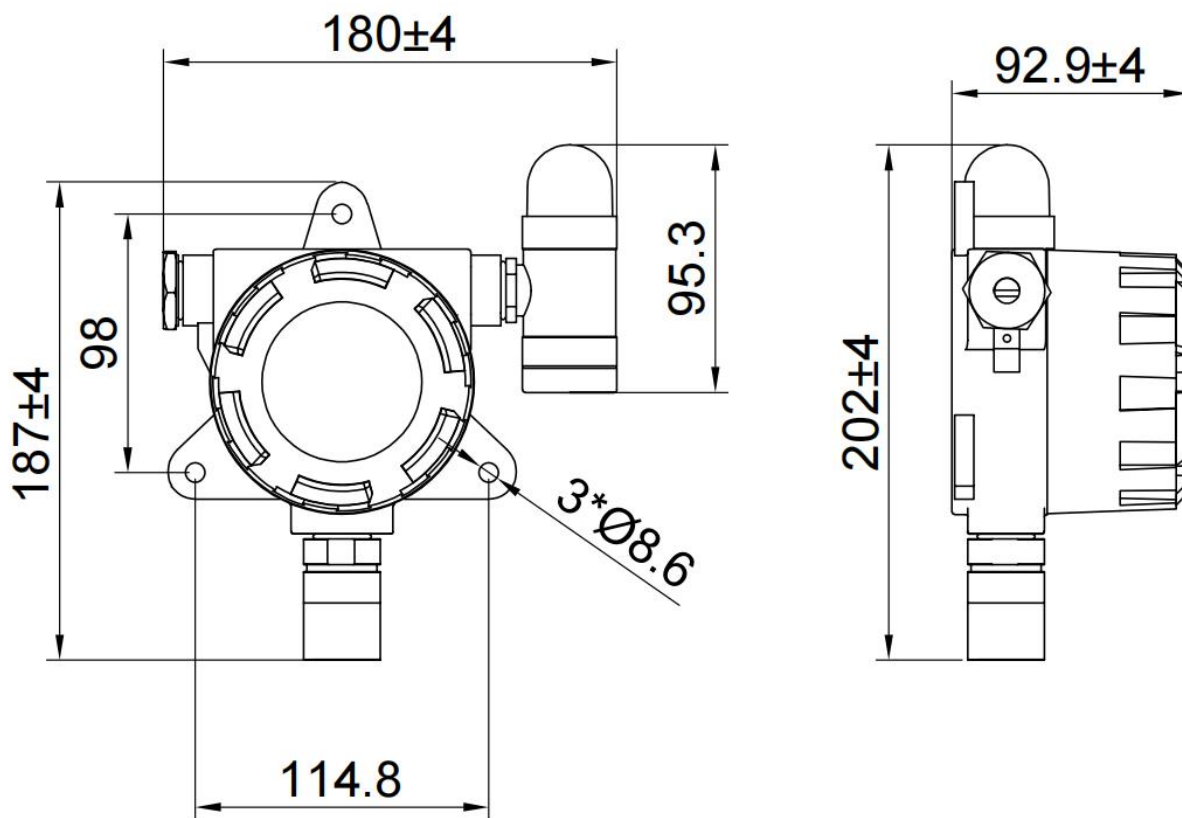
带声光报警器壳体尺寸图（单位：mm）
