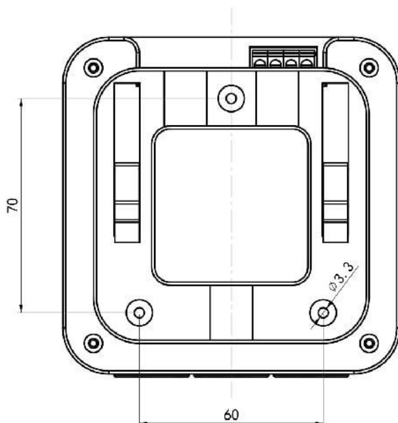
安装底座尺寸（单位：mm）
