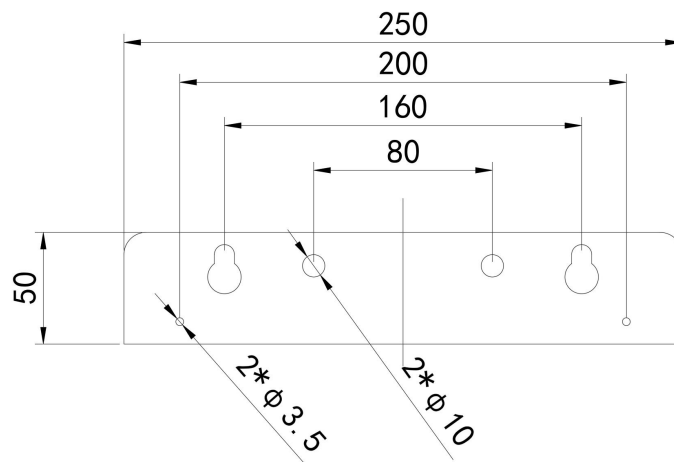
安装板尺寸 (单位 mm)
