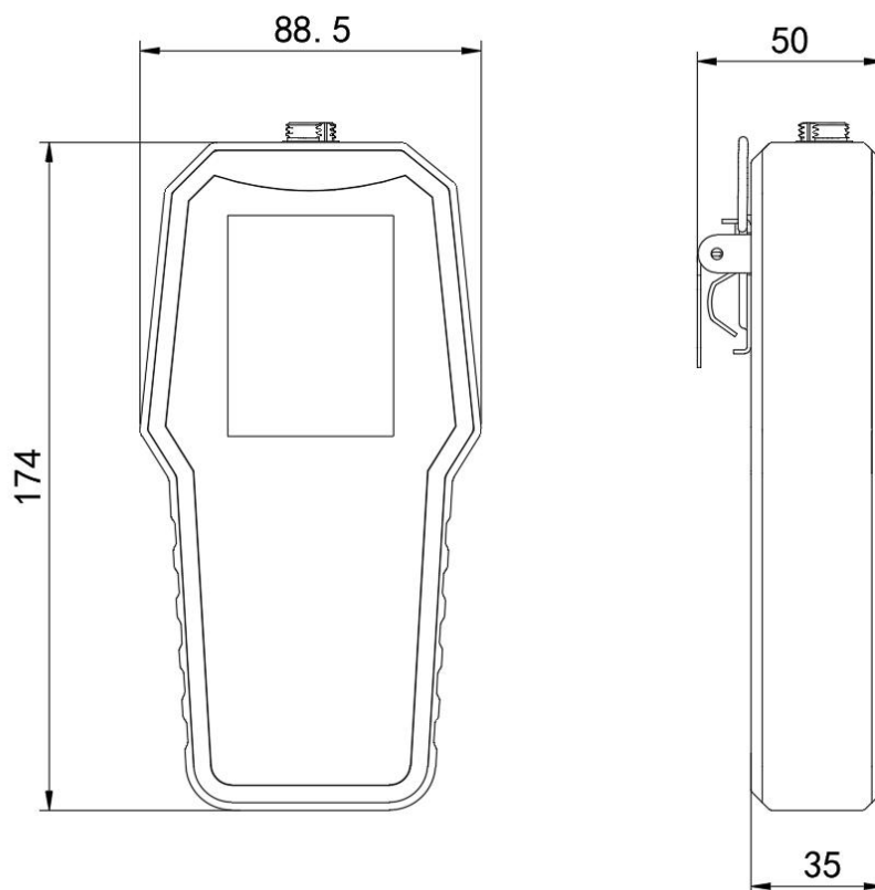
设备尺寸图（单位：mm）
