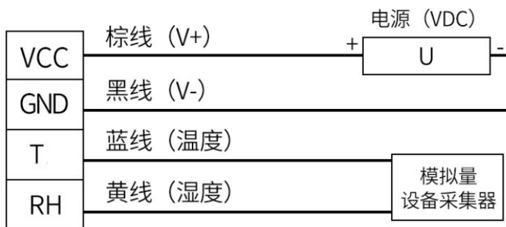
模拟量接线示意图
