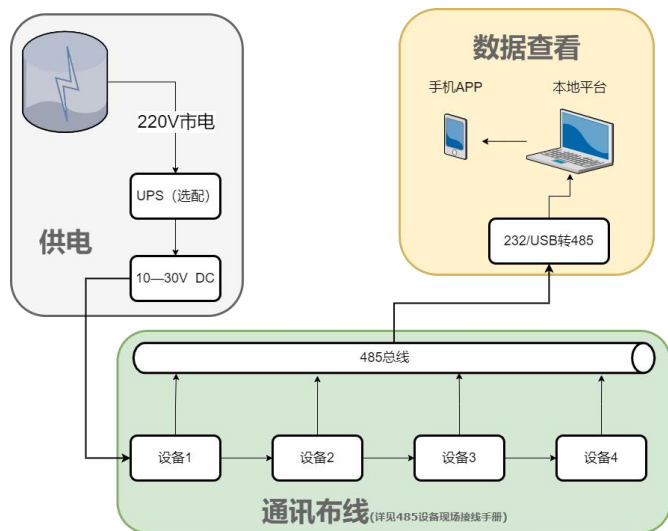
485 设备使用拓扑图
