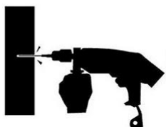
1 用钻头在墙壁上钻孔 孔径12mm 孔距160mm
