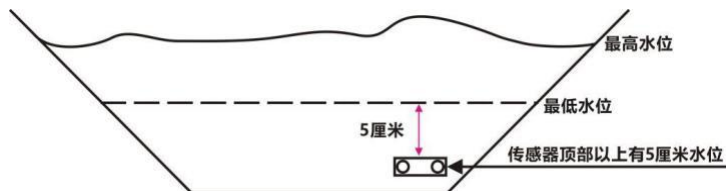
多普勒流速仪安装在梯形渠道的“坡脚”
