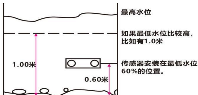
多普勒流速仪安装在最低水位一半的位置
