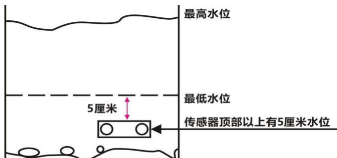
多普勒流速仪顶部以上要有至少 5 厘米的水位
