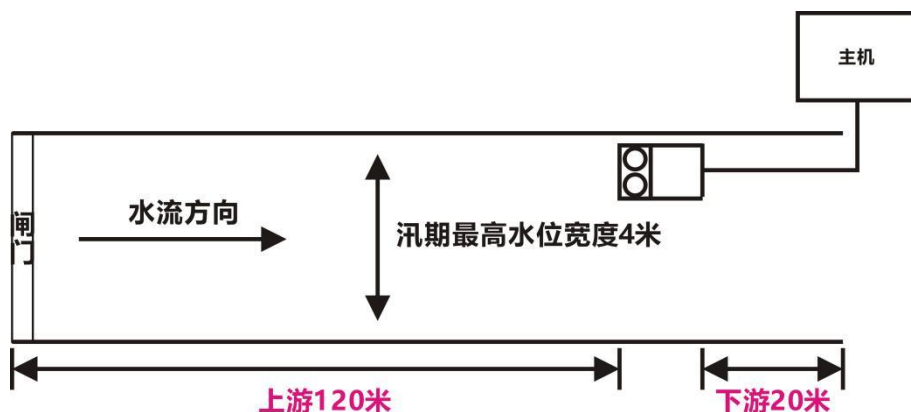
在闸门下游安装对直渠道长度要求
