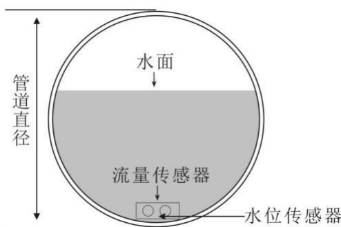
无沉积物管道的安装位置
