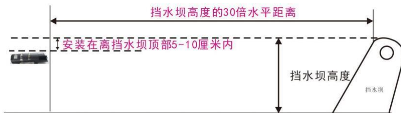
装在靠近挡水坝顶部的位置
