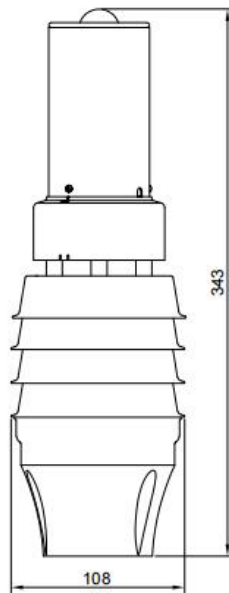
-3HP 设备尺寸（单位 mm）
