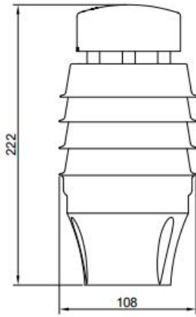
-3H 设备尺寸图（单位：mm）
