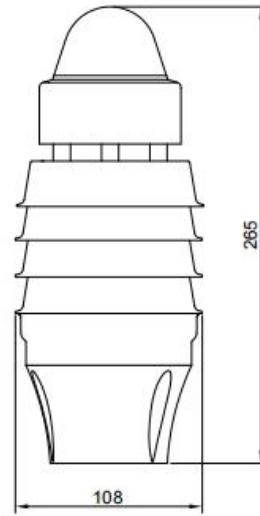
-3H 带光学雨量要素尺寸图（单位：mm）
