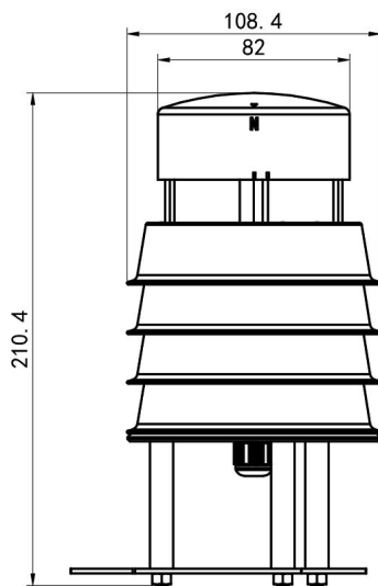
-3 设备尺寸图（单位 mm）
