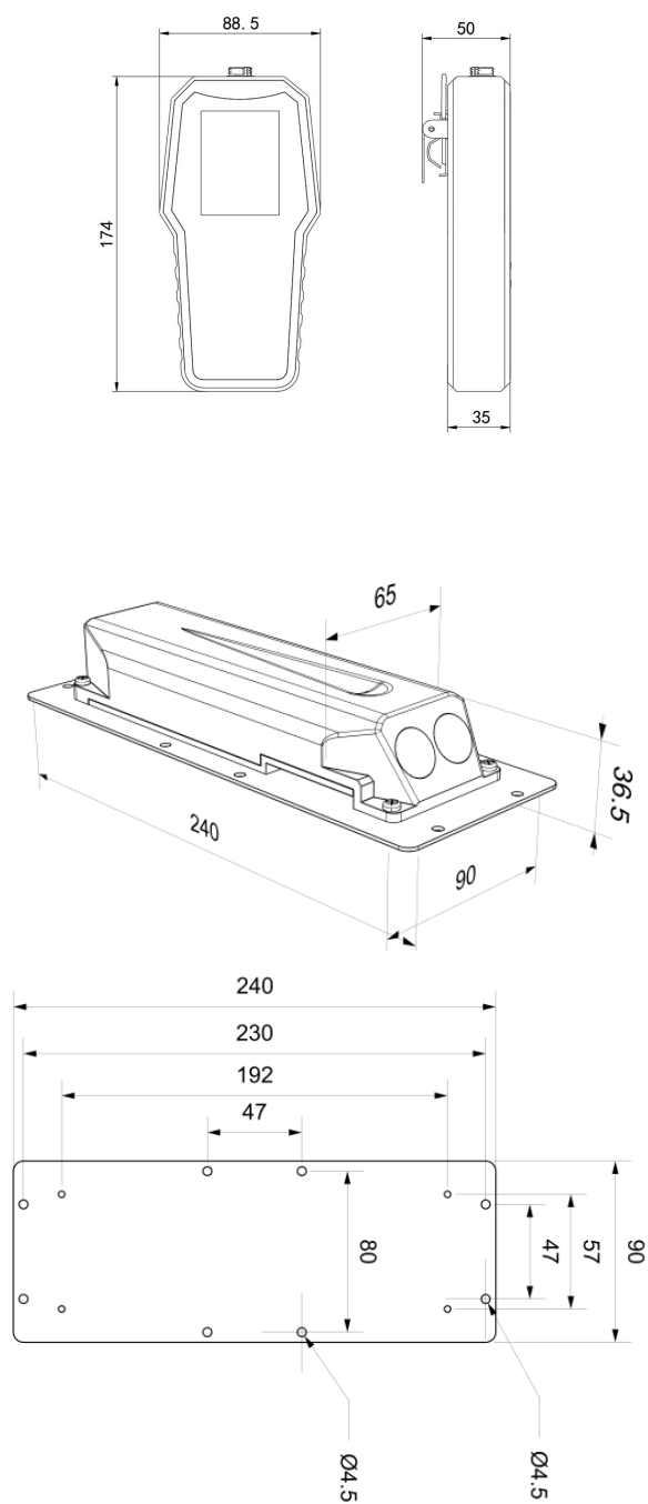
设备尺寸图（单位：mm）
