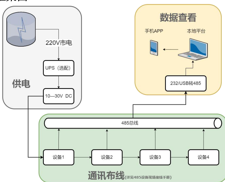
485 设备使用拓扑图
