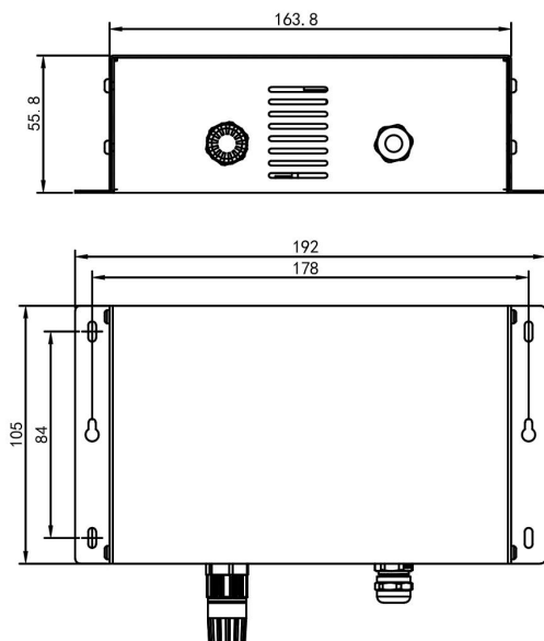
尺寸图（单位：mm）
