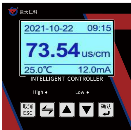
电导率测量模式界面
