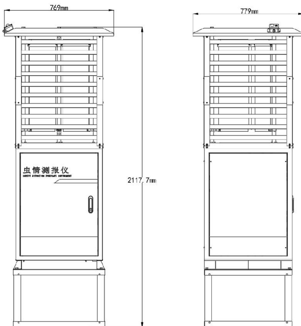
安装尺寸（单位：mm）
